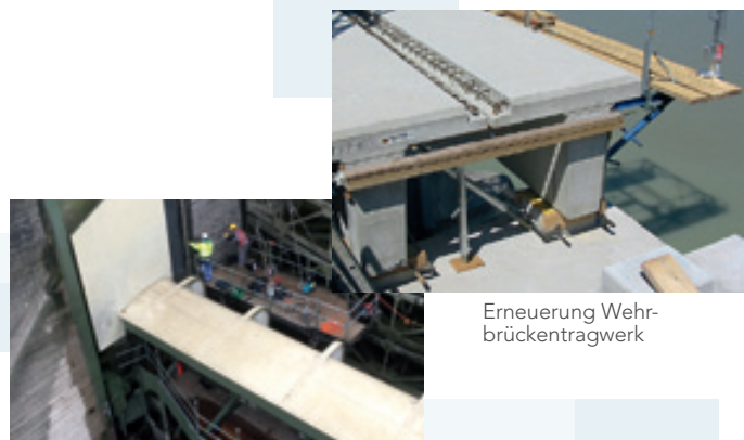
Betoninstandsetzung im Wehrfeld
